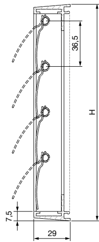
Technologie Renson® grille de hotte 433/S
