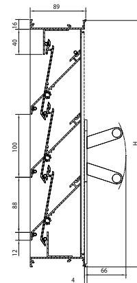
Zonder flens nr. 427ZF
