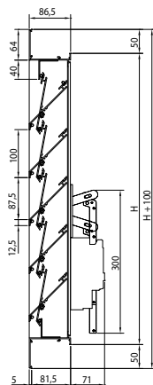
Type 427/4 Motorbediening 220 Volt - 24 Volt Minimumhoogte van het rooster 390 mm
